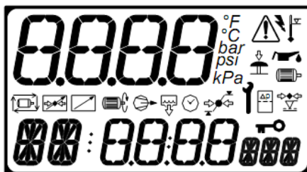
Рис. 1. Дисплей контроллера
