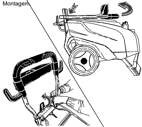
Montagem
