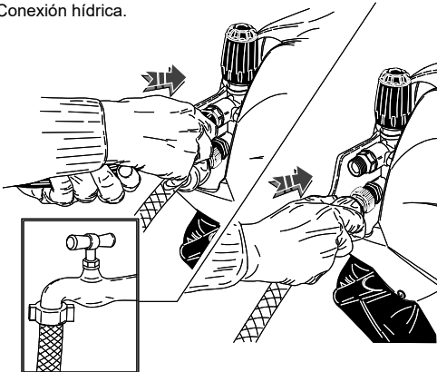
Conexión hídrica.
