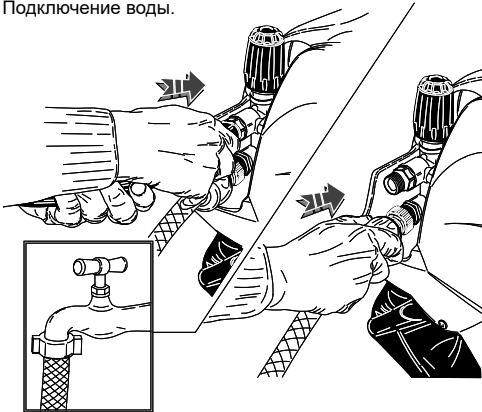
Подключение воды.
